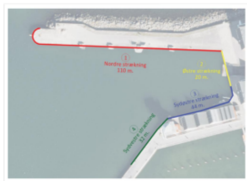
Strækningsoversigt
